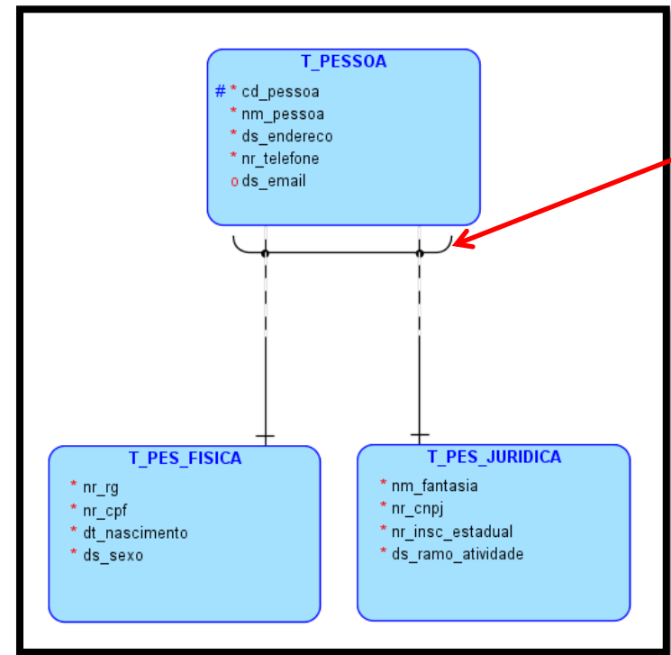
Notação: Barker
